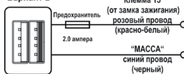
рис.2 Схема подключения
