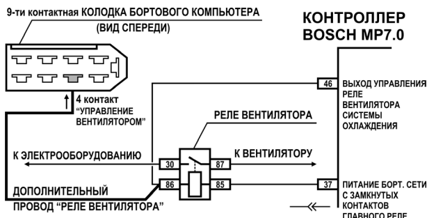
рис. 4 Аппаратное подключение функции «ТРОПИК»
