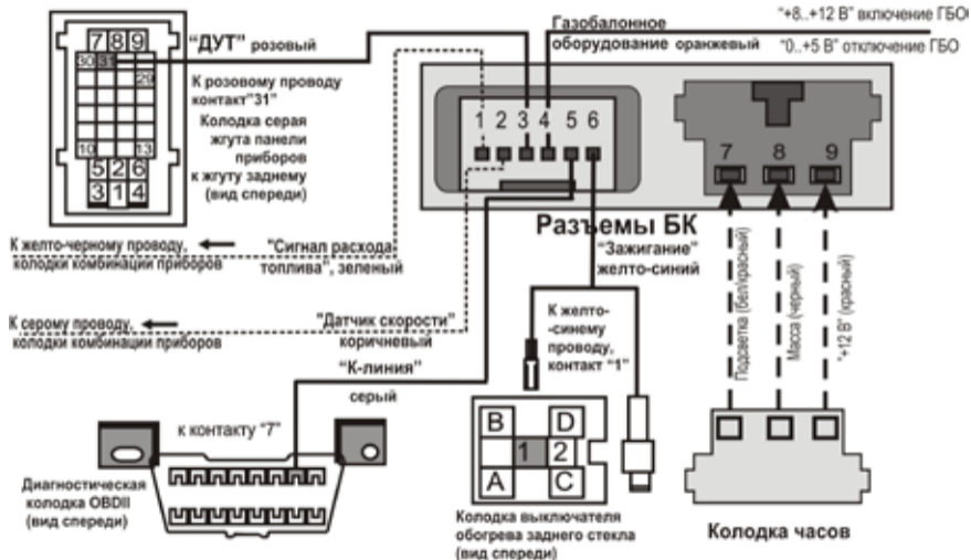
Рис. 8 Схема подключения
