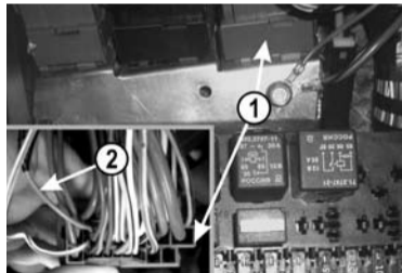
Рис. 9 Подключение сигнала ДУТ
