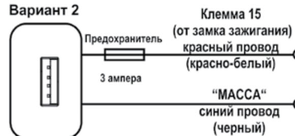
рис.2 Схема подключения
